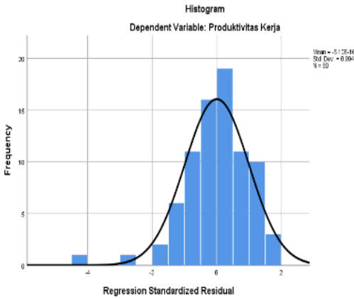
Gambar 1. Uji Normalitas
