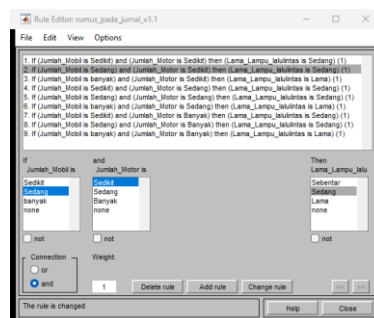
Gambar 5. Editor Aturan Fuzzy
