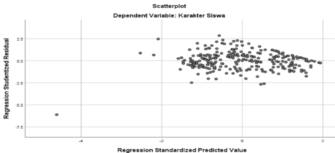
Gambar 2. Uji heteroskedastisitas
