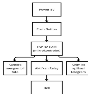
Gambar 2. Blok Diagram Sistem
