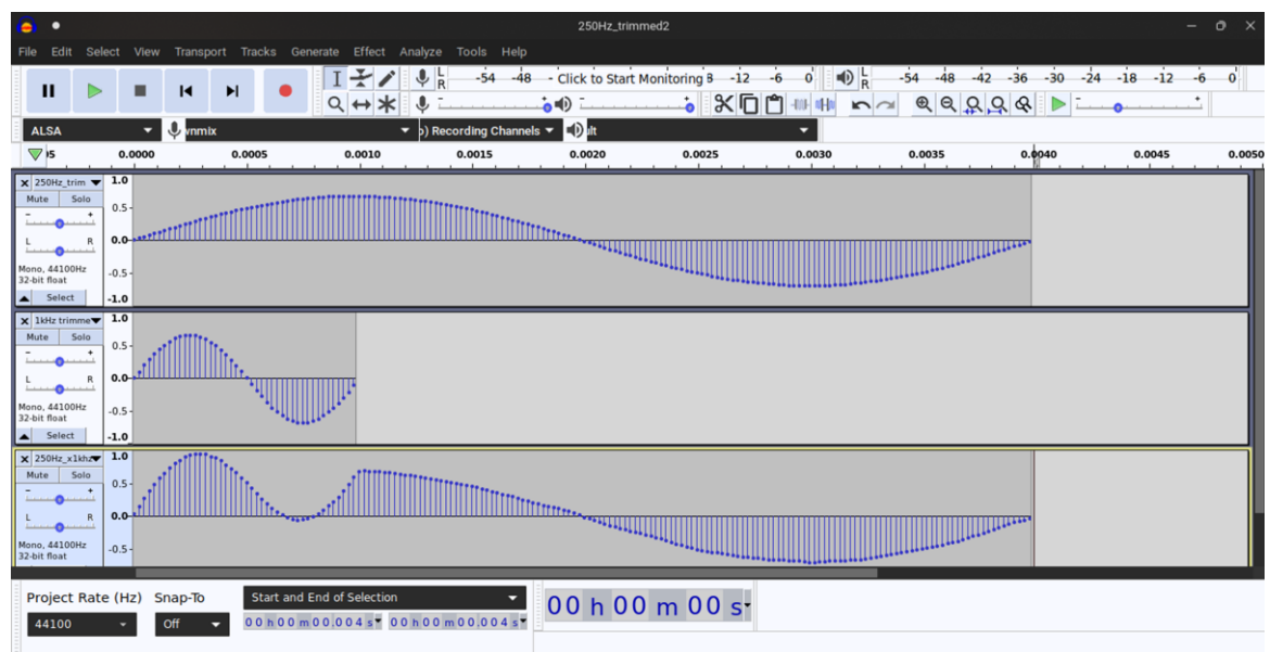
Gambar 4. Hasil superposisi gelombang 250 Hz vs 1 kHz
