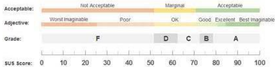
Gambar 17 Penentuan Hasil Penilaian Skor SUS
