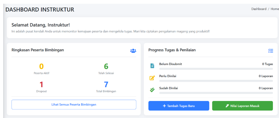
Gambar 8. Instruktur Dashboard
