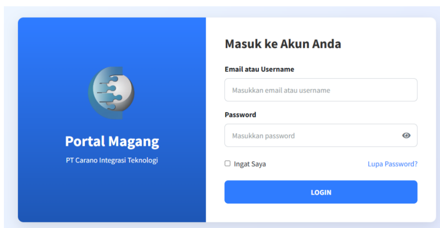
Gambar 3. Halaman Login
