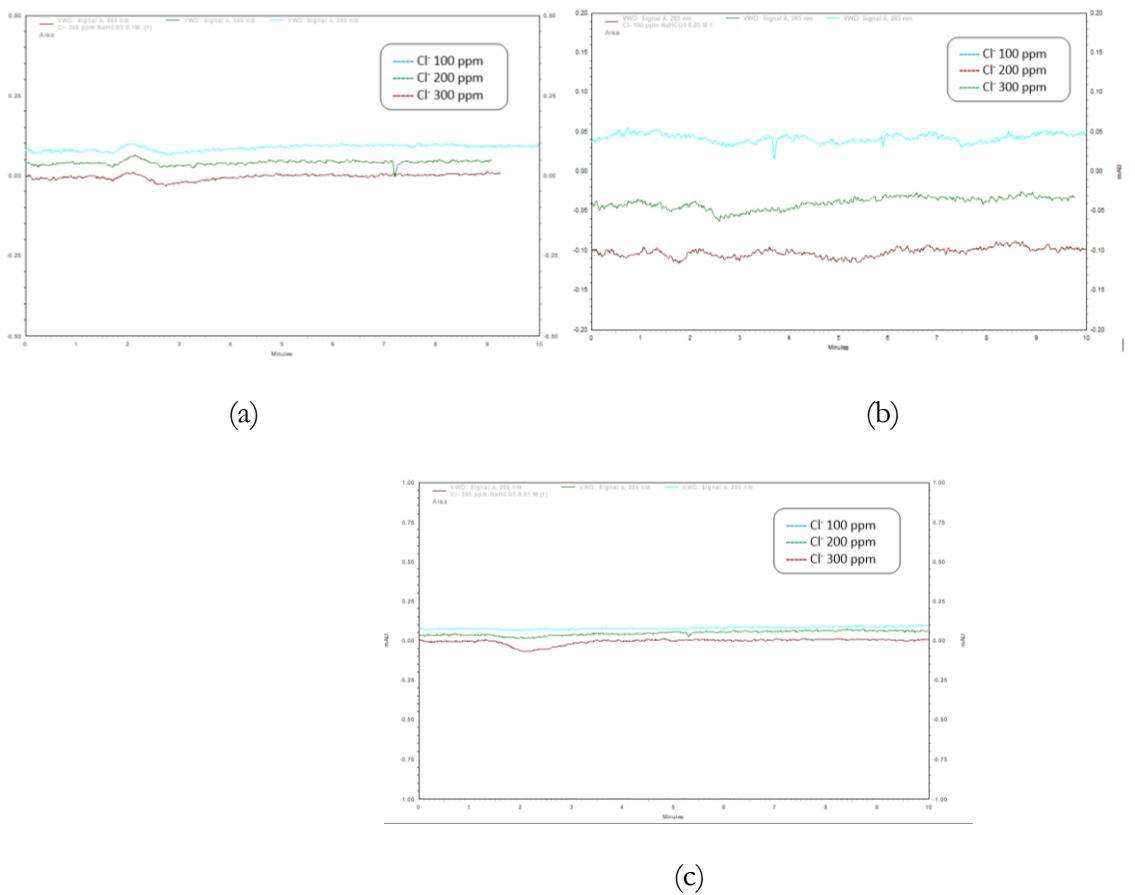
Gambar 4. Kromatogram ion Klorida (a) NaHCO 3 0,1 M (b) NaHCO 3 0,05 M (c) NaHCO 3 0,01 M
