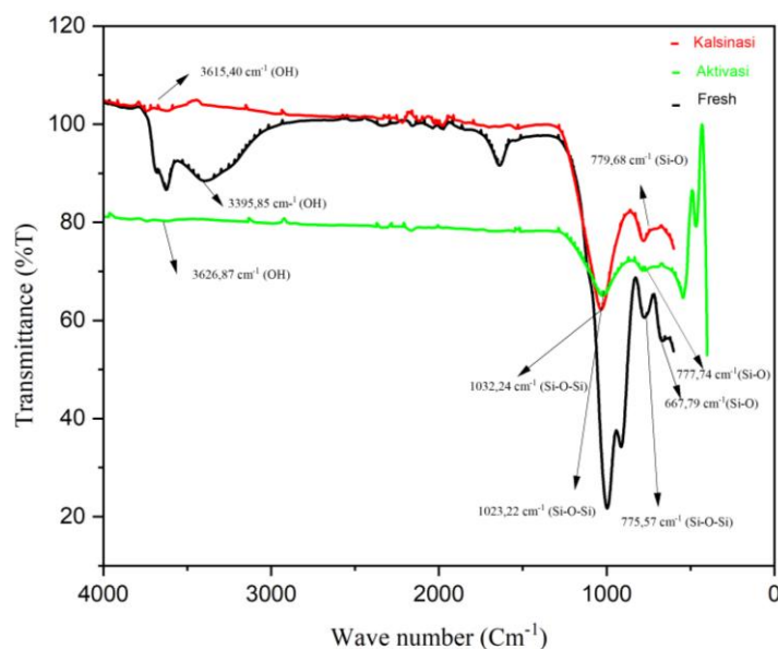
Gambar 1. Karakterisasi FTIR tanah napa
