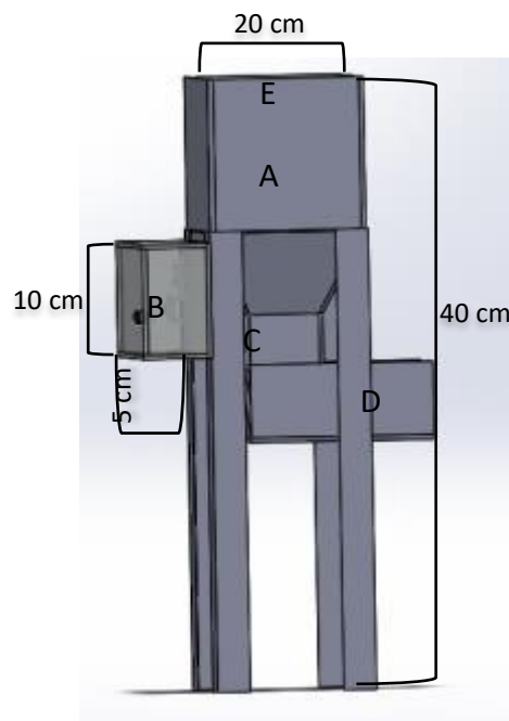
Gambar 4. Desain 3D
