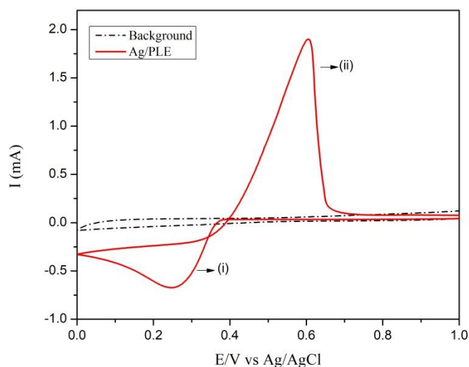
Gambar 1. Voltammogram siklik elektrodposisi modifikasi PLE dalam 5 Mm \text{AgNO}_3 dan 0,1 M \text{KNO}_3 dengan scan rate 100 mV/s.
