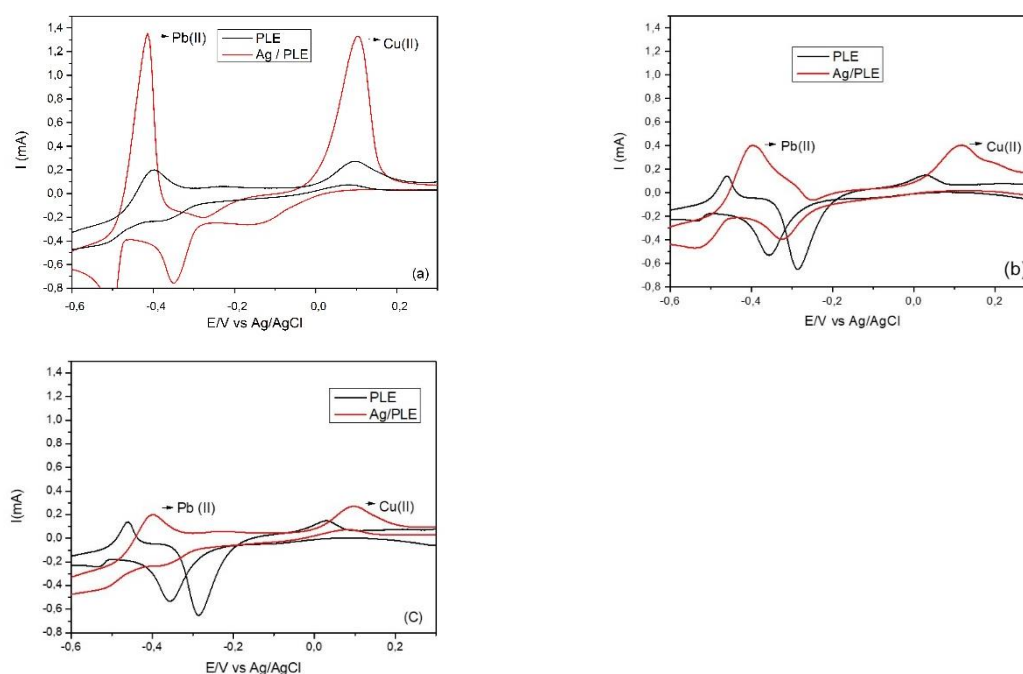
Gambar 2. Voltammogram siklik pada Ag/PLE dalam variasi supporting electrolyte (a) \text{HNO}_3 0,1 M, (b) \text{HCl} 0,1 M, (c) \text{H}_2\text{SO}_4 0,1 M scan rate 100 mV/s.
