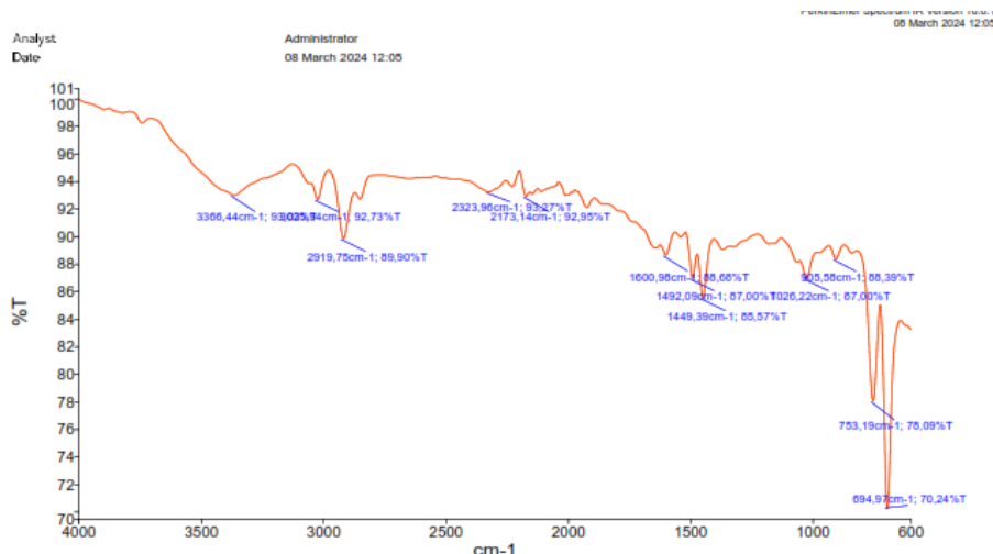
Gambar 2. Spektrum FTIR sampel tertutup
