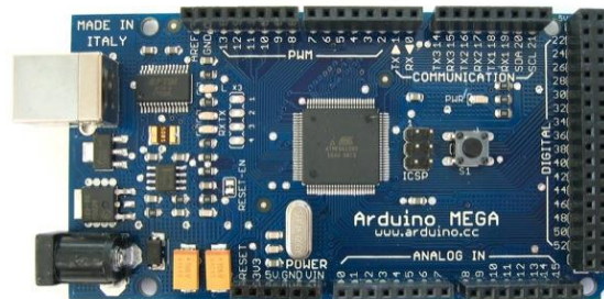
Gambar 3. Arduino mega 2560
