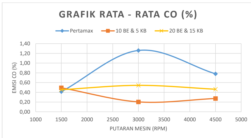
Gambar 3 Grafik Hasil Rata – Rata Gas CO
