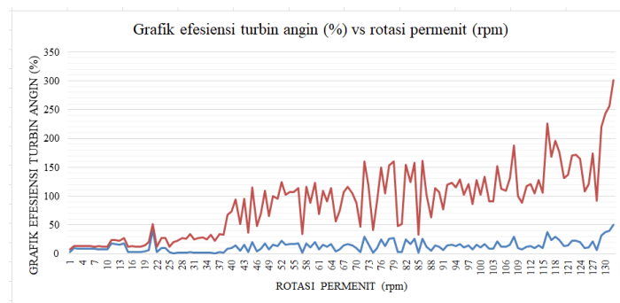
Gambar 9 Grafik Hubungan Efesiensi Turbin Angin Terhadap Rotasi Permenit
