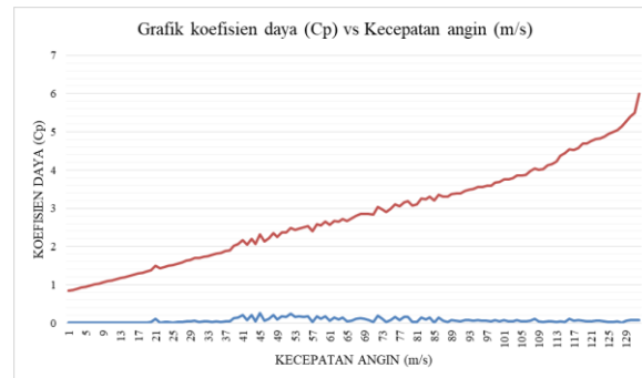
Gambar 3 Grafik Hubungan Koefisien Daya Terhadap Kecepatan Angin
