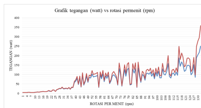
Gambar 2 Grafik Hubungan Tension Terhadap Rotasi Permenit
