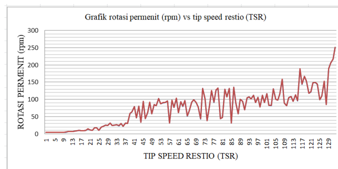
Gambar 11. Grafik Hubungan Rotasi Permenit Terhadap Tip Speed Restio
