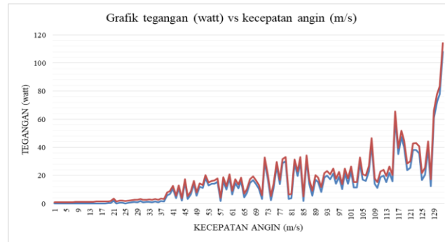
Gambar 5 Grafik Hubungan Tension Terhadap Kecepatan Angin
