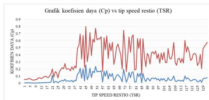
Gambar 7 Grafik Hubungan Koefisien Daya Terhadap Tip Speed Restio
