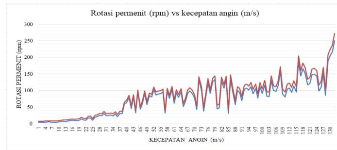
Gambar 10 Grafik Hubungan Rotasi Permenit Terhadap Kecepatan Angin
