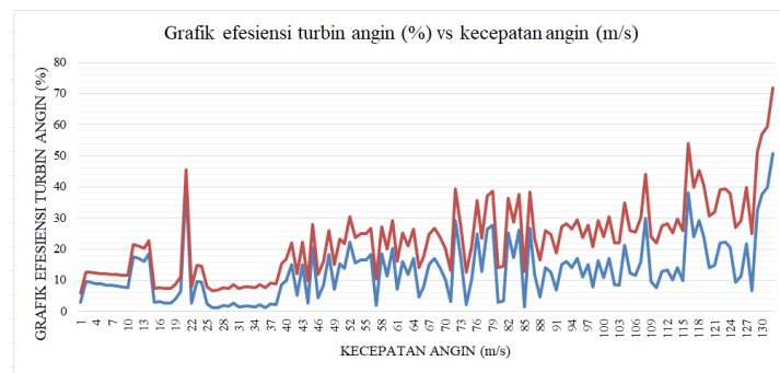
Gambar 6 Grafik Hubungan Efisiensi Turbin Angin Terhadap Kecepatan Angin
