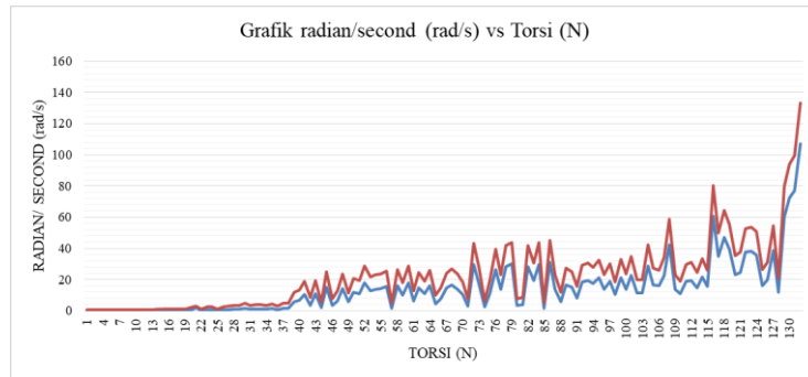
Gambar 8 Grafik Hubungan Radian/Second Terhadap Torsi
