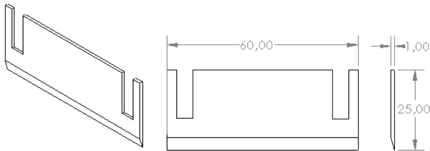
Gambar 4. Bilah mata pisau
