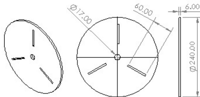
Gambar 2. Dudukan dengan 3 mata pisau
