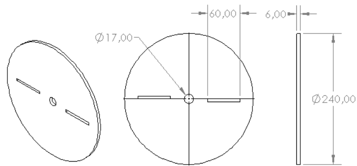
Gambar 1. Dudukan dengan 2 mata pisau
