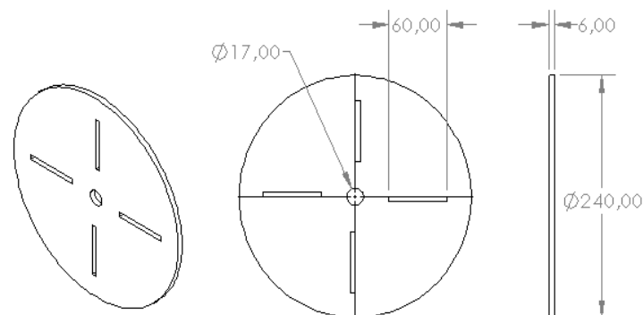
Gambar 3. Dudukan dengan 4 mata pisau
