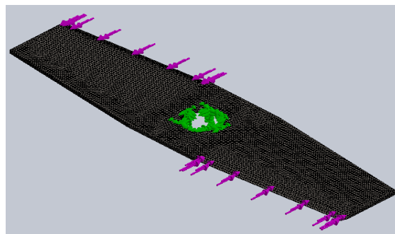
Gambar 5. Visualisasi Meshing
