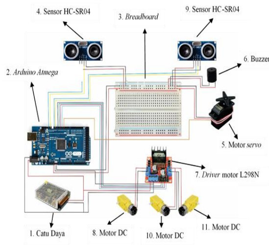
Gambar 2 Desain komponen elektronika
