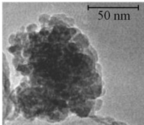
Gambar 13 Morfologi TEM dari nanopartikel \text{TiO}_2 dengan metode sonokimia (Arami et al., 2007).
