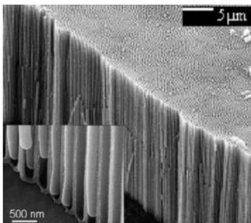
Gambar 12 Morfologi SEM cross-sectional dari kawat nano \text{TiO}_2 elektrodeposisi dalam pori-pori AAM (Liu et al., 2013)
