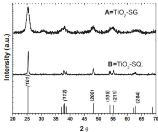
Gambar 7 Pola difraksi sinar-X dengan metode sol-gel (Ángel-sanchez et al., 2013).
