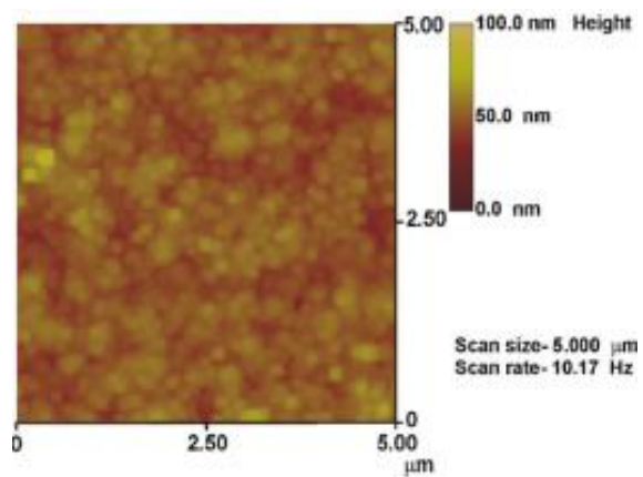
Gambar 11 Analisis Atomic Force Microscopy (AFM) lapisan tipis TiO 2 dengan metode deposisi uap kimia (suhu 400°C) (Shinde & Bhosale, 2008).
