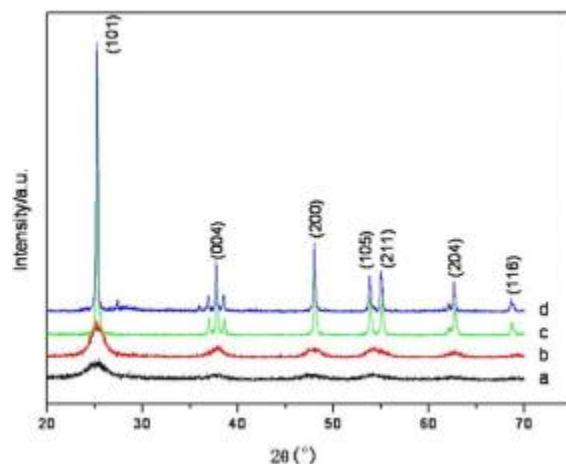
Gambar 16 Pola difraksi sinar-X nanopartikel TiO 2 dengan metode gelombang mikro (X. Wu et al., 2005).
