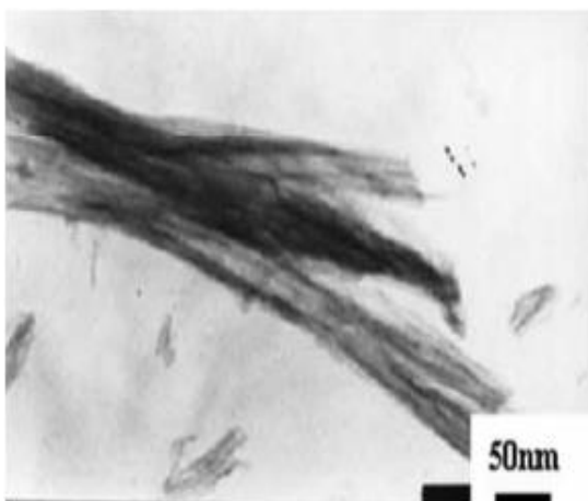
Gambar 15 Morfologi TEM dari tabung nano TiO 2 dengan metode gelombang mikro (X. Wu et al., 2005).
