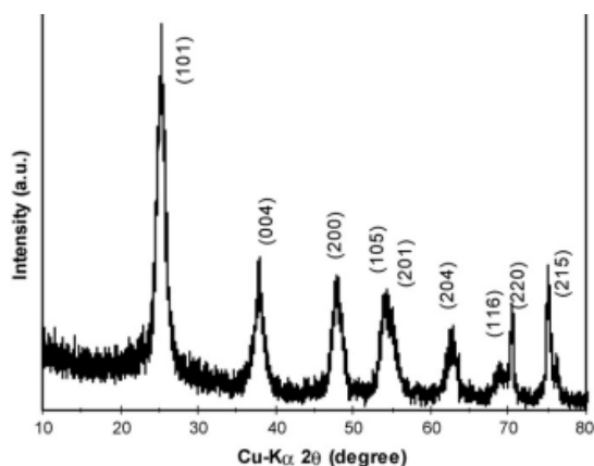
Gambar 3 Pola difraksi sinar-X \text{TiO}_2 anatase mesopori (Pavasupree et al., 2008)
