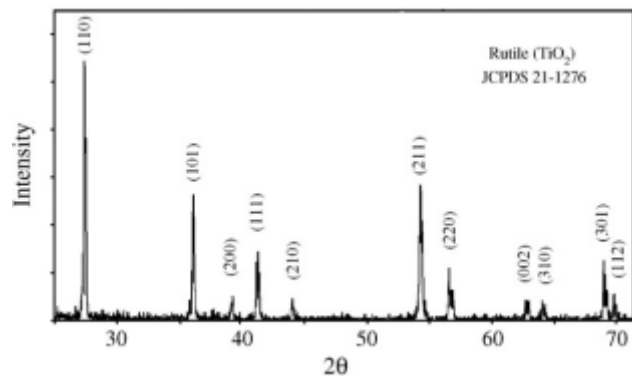
Gambar 14 Pola difraksi sinar-X nanopartikel \text{TiO}_2 dengan metode sonokimia (Arami et al., 2007).
