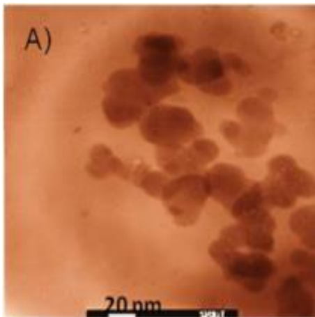
Gambar 6 Morfologi TEM \text{TiO}_2 dengan metode sol-gel dan kalsinasi pada suhu 400^\circ\text{C} (Ángel-sanchez et al., 2013).
