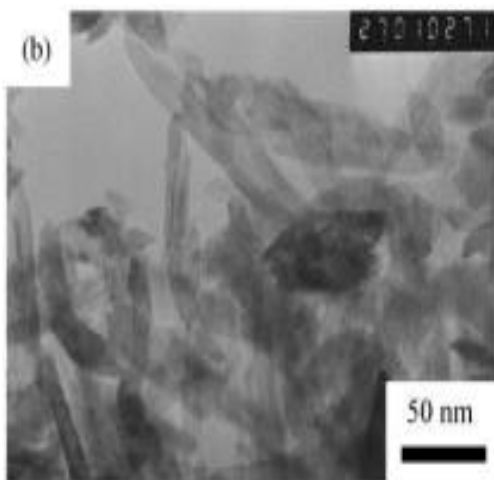
Gambar 8 Morfologi TEM nanorods TiO 2 dengan metode oksidasi langsung pelat Ti dengan larutan H 2 O 2 (J. Wu, 2004).
