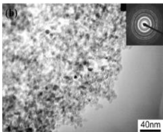
Gambar 2 Morfologi TEM partikel nano \text{TiO}_2 dengan metode hidrotermal (Pavasupree et al., 2008)
