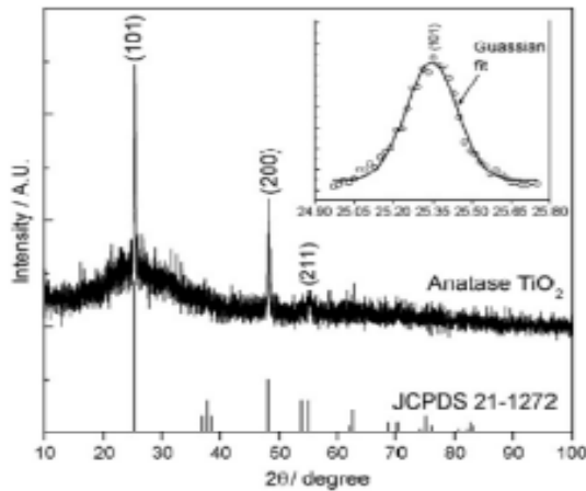
Gambar 10 Pola difraksi sinar-X endapan uap kimia (suhu penguapan 400°C) lapisan tipis TiO 2 anatase pada kaca soda kapur (Shinde & Bhosale, 2008).
