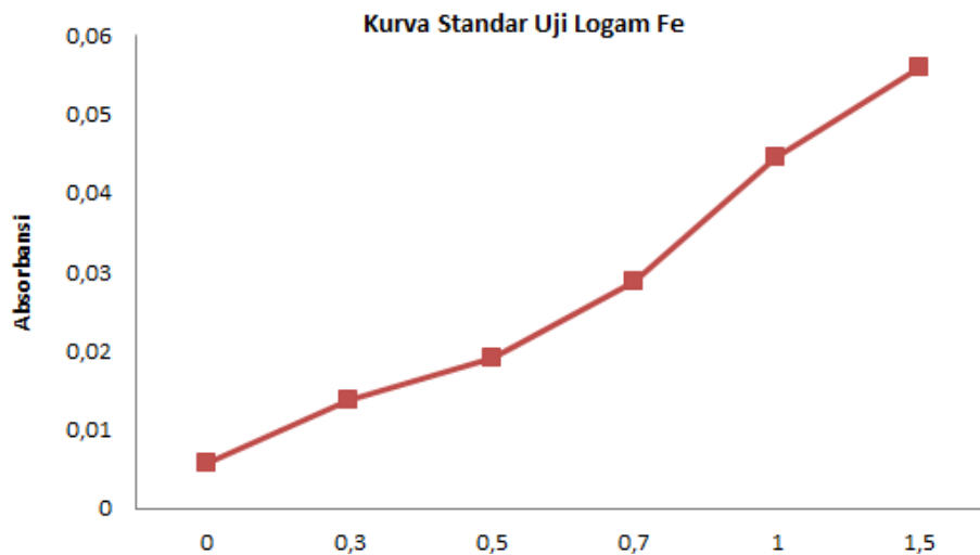
Grafik 1. Kurva Standar Uji Logam Fe
