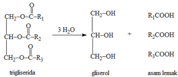
Gambar 3. Reaksi hidrolisis trigliserida
