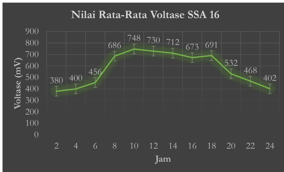
Gambar 2. Grafik pengukuran Voltase
