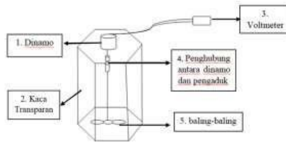
Gambar 2. Desain reaktor
