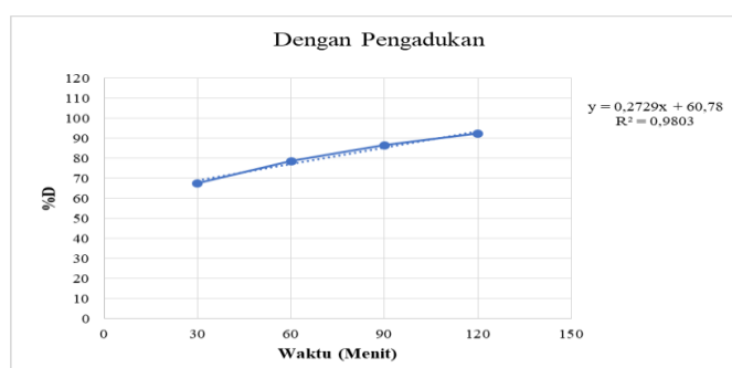
Gambar 3. Grafik degradasi methylene blue dengan pengadukan
