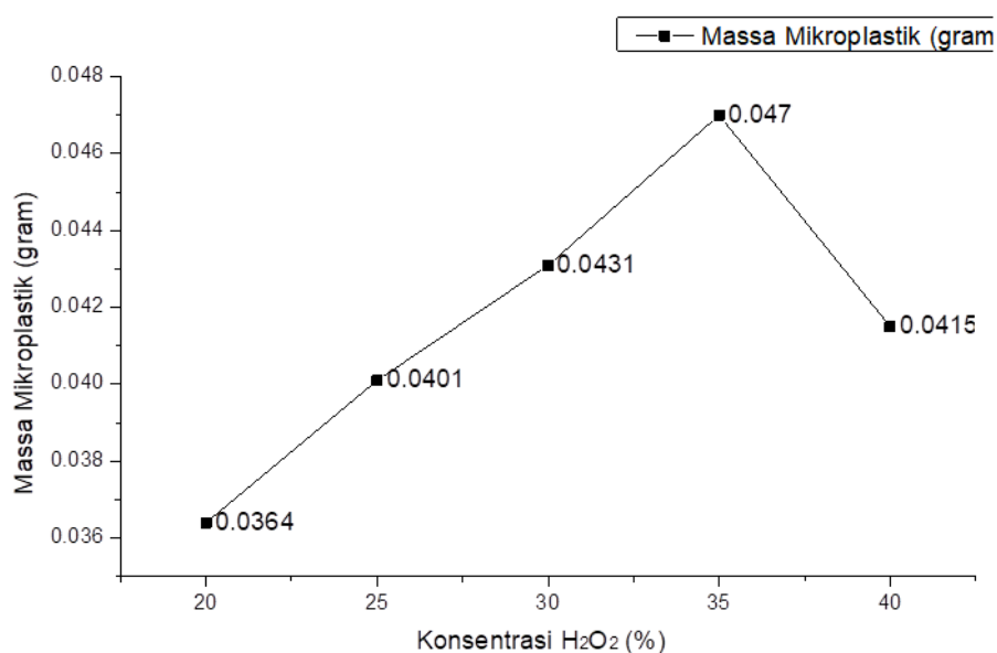
Gambar 3. Grafik Variasi Konsentrasi H_2O_2
