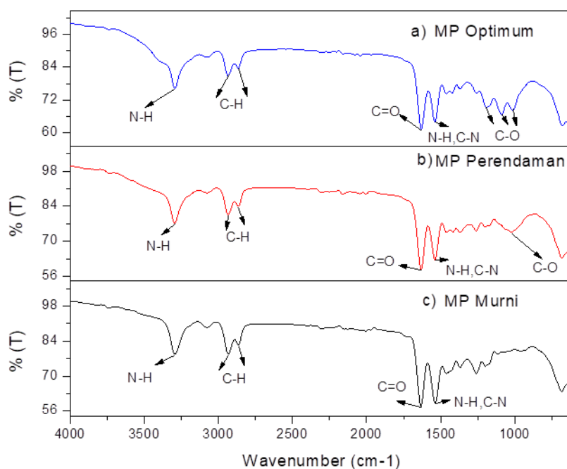
Gambar 4. Spektrum Fourier Transform Infra Red (FTIR) Mikroplastik Poliamida (PA). a) Mikroplastik Optimum, b) Mikroplastik Perendaman, c) Mikroplastik Murni
