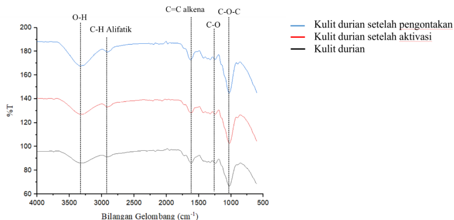
Gambar 1. Spektrum FTIR serbuk kulit durian, serbuk kulit setelah durian aktivasi, serbuk kulit durian setelah pengontakan.
