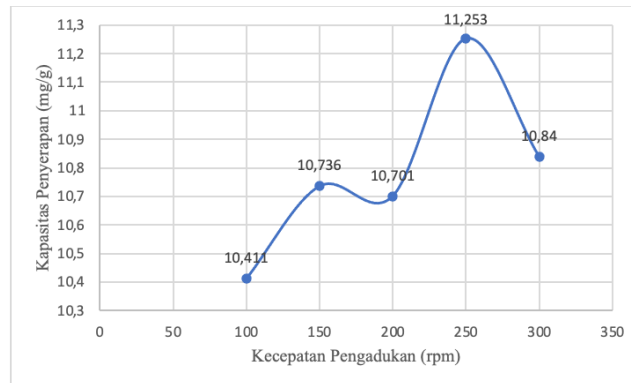
Gambar 2. Grafik pengaruh Kecepatan Pengadukan terhadap kemampuan retensi partikel logam \text{Cu}^{2+} dengan serbuk kulit durian
