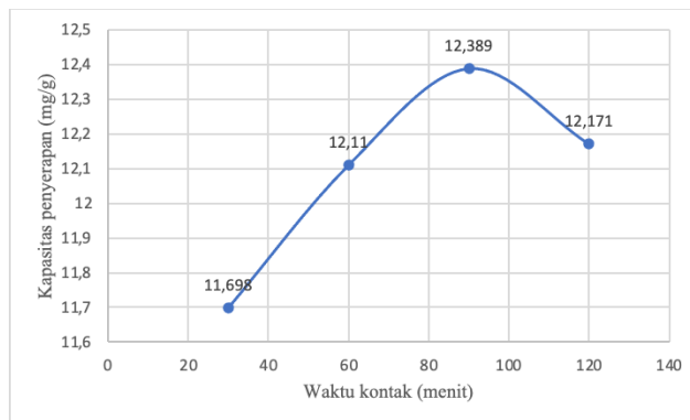
Gambar 3. Grafik pengaruh Waktu Kontak terhadap kemampuan retensi partikel logam \text{Cu}^{2+} dengan serbuk kulit durian
