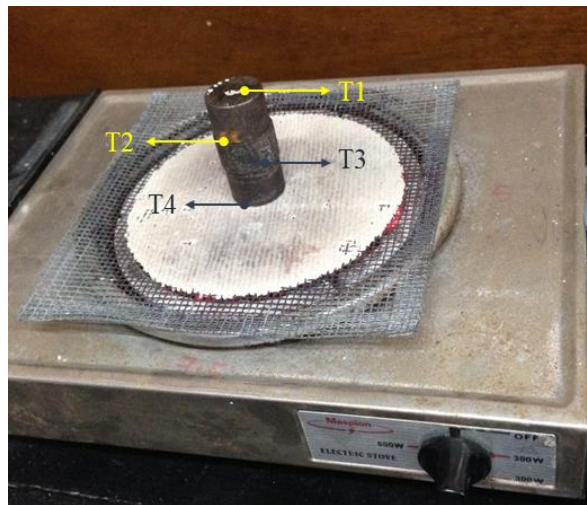
Gambar 2. Proses pemanasan material yang diukur konduktivitasnya
