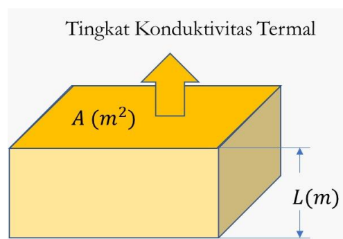
Gambar 1. Mekanisme Konduktivitas Termal
