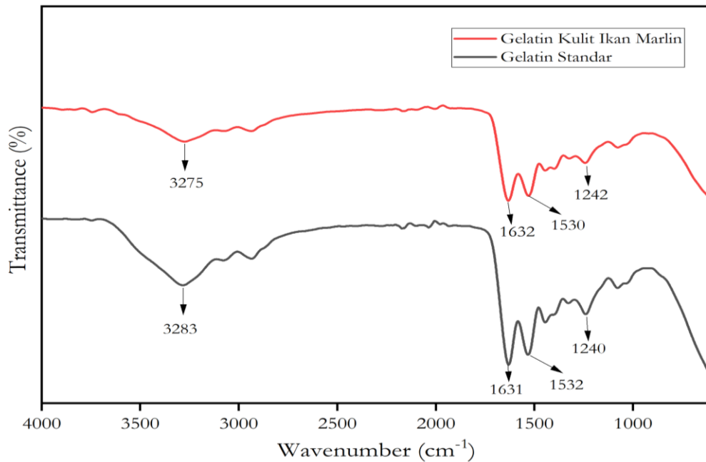
Gambar 1. Spektrum FTIR Gelatin Kulit Ikan Marlin dengan Gelatin Standar
