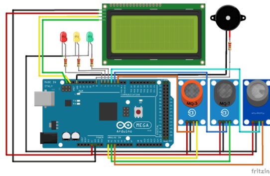
Gambar 9. Rangkaian Arduino Mega 2560
