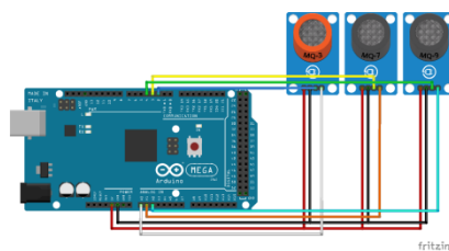
Gambar 10. Rangkaian Sensor Gas
