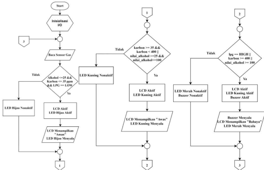
Gambar 14. Flowchart Arduino Mega 2560
