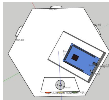
8. Rancangan Tampilan Atas
