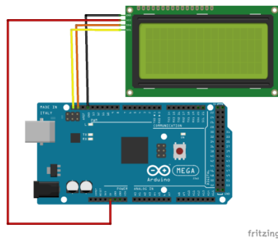
Gambar 11. Rangkaian LCD 20x4 I2C
