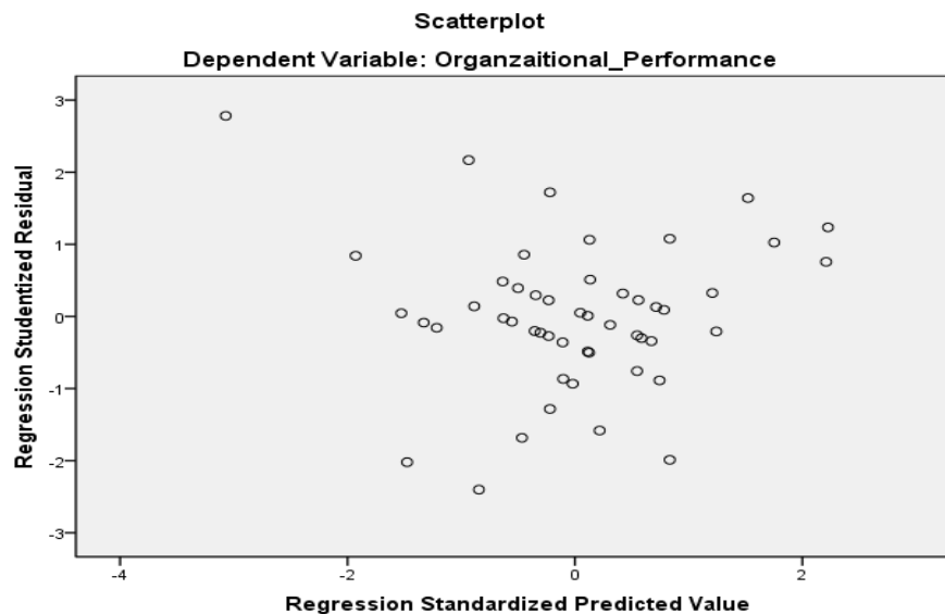
Gambar 2. Pengujian Heteroskedastisitas dengan Grafik Scatterplot
