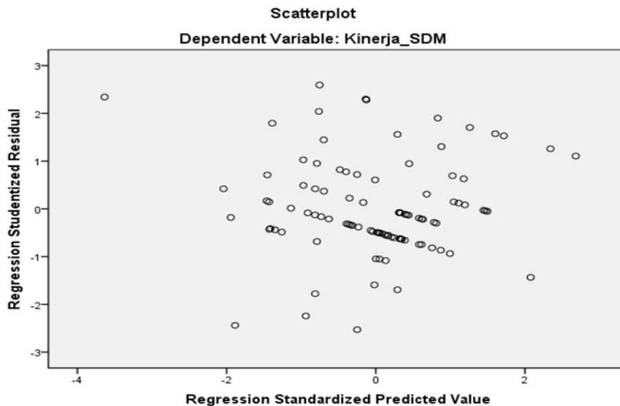
Gambar 1. Pengujian Normalitas dengan Grafik Scatterplot
