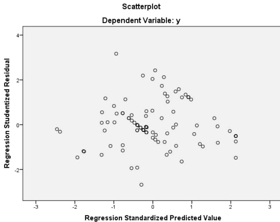
Gambar 2. Uji Heteroskedastitas
