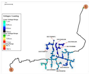
Gambar 6. Analisa Tegangan Jatuh Pola Operasi 2
