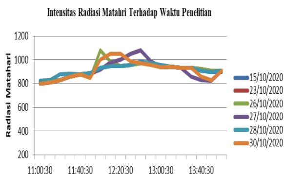
Gambar 3. Intensitas Radiasi Matahari Terhadap Waktu Pengambilan Data
