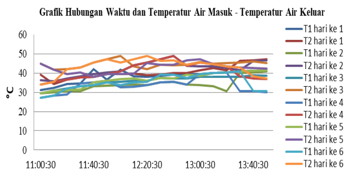
Gambar 4. Temperatur Air Masuk dan Air Keluar Pengujian Solar Heater
