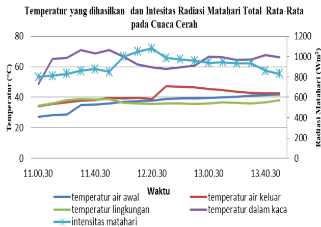
Gambar 5. Grafik Temperatur Kondisi Pengujian Cuaca Cerah
