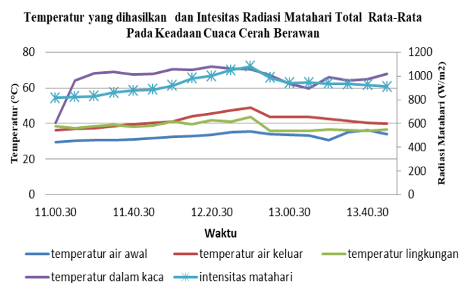
Gambar 6. Grafik Temperatur Kondisi Pengujian Cuaca Cerah Berawan
