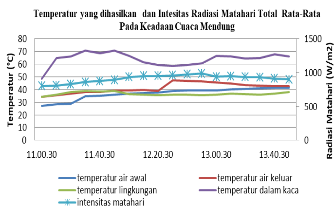
Gambar 7. Grafik Intesitas Dan Temperatur Cuaca Mendung
