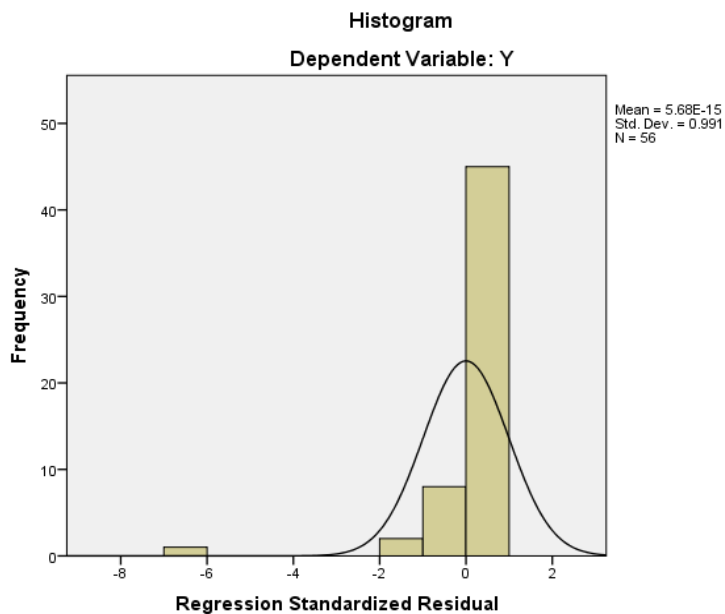
Gambar 1 Grafik Pengujian Normalitas Data
