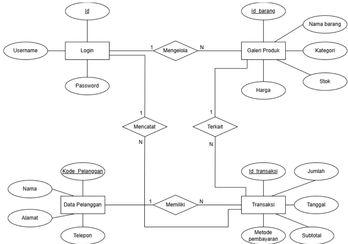
Gambar 2 ERD
