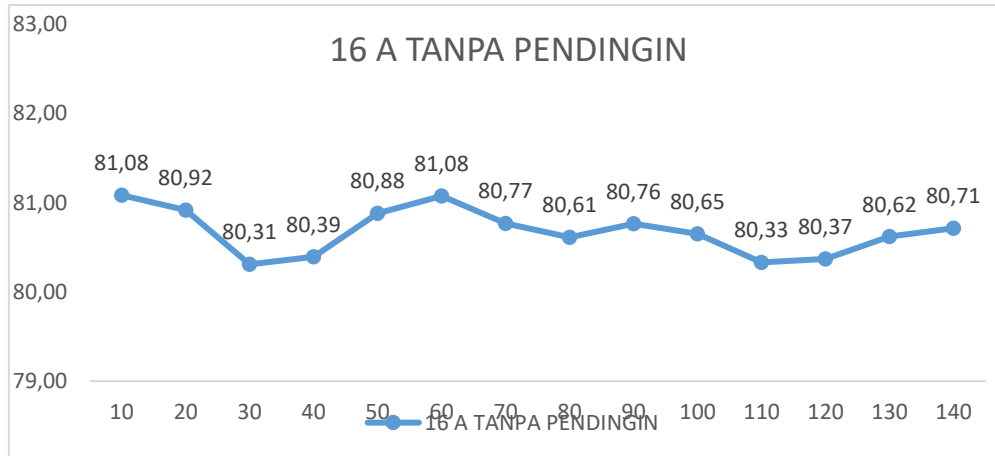
Gambar 8 Grafik Nilai Tegangan Masuk saat Arus 16 A Tanpa Pendingin
