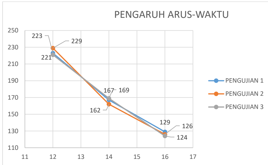
Gambar 9. 1 Grafik Pengaruh Arus dan Waktu
