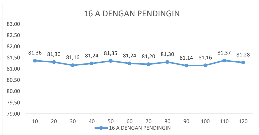
Gambar 7 Grafik Nilai Tegangan Masuk saat Arus 16 A Dengan Pendingin
