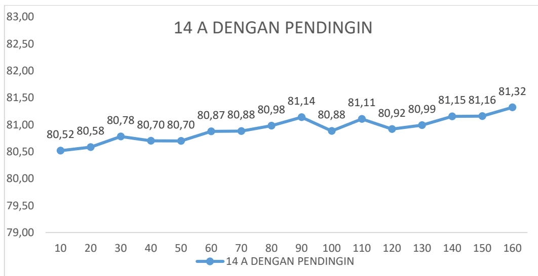
Gambar 5 Grafik Nilai Tegangan Masuk saat Arus 14 A Dengan Pendingin
