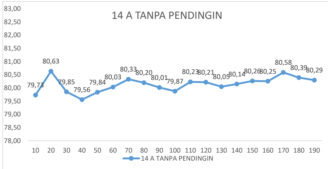
Gambar 6 Grafik Nilai Tegangan Masuk saat Arus 14 A Tanpa Pendingin
