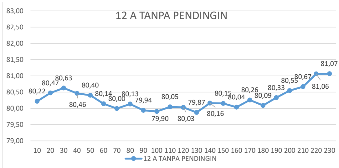
Gambar 4 Grafik Nilai Tegangan Masuk saat Arus 12 A Tanpa Pendingin
