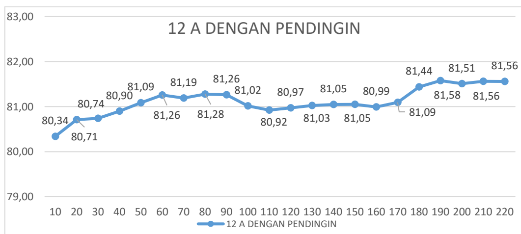
Gambar 3 Grafik Nilai Tegangan Masuk saat Arus 12 A Dengan Pendingin
