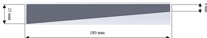
Gambar 3 Desain dan ukuran pasak pada crossbar.
