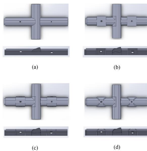
Gambar 2 Desain original ( a), modifikasi 1 (b), modifikasi 2 (c), modifikasi 3 (d).
