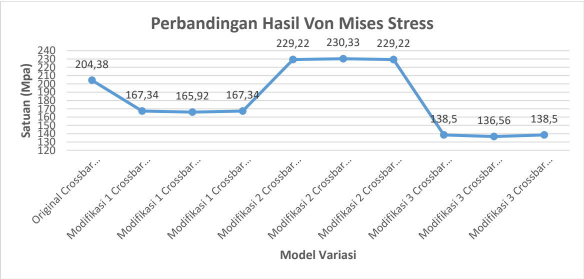
Grafik 1 Perbandingan hasil analisa tegangan (Von Mises) stress
