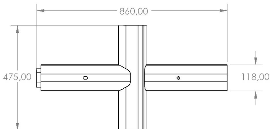
Gambar 1 Desain utama komponen crossbar clinker cooler.
