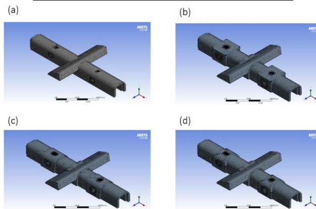
Gambar 4 Meshing Original, (b) meshing modifikasi 1, (c) meshing modifikasi 2, (d) meshing modifikasi 3.
