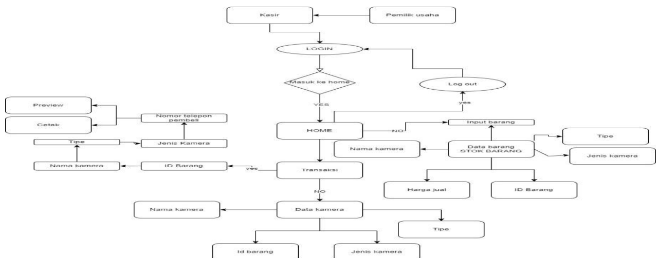
Gambar 2 . ERD
