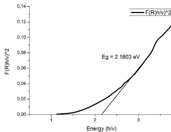
Gambar 3. Grafik Bandgap \text{CuSnO}_3 0,075 M
