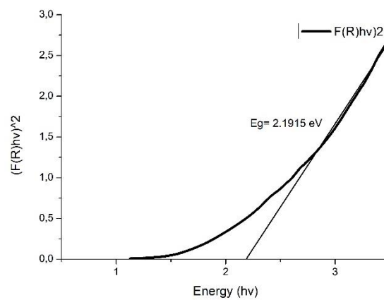
Gambar 2. Grafik Bandgap \text{CuSnO}_3 0,05 M
