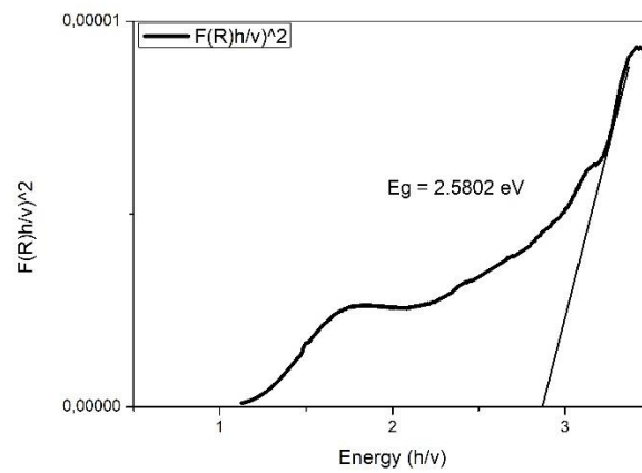
Gambar 1. Grafik Bandgap \text{CuSnO}_3 0,025 M
