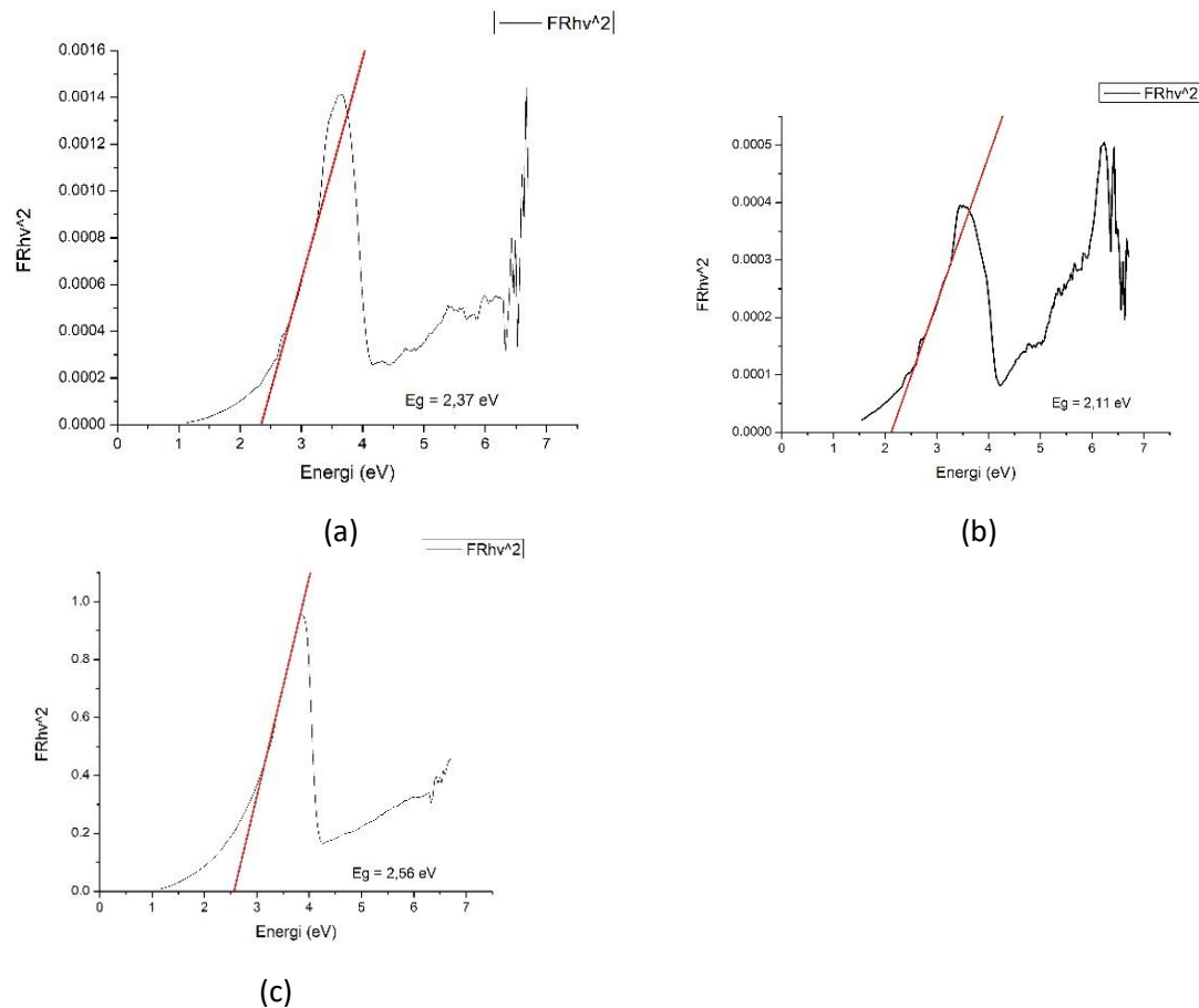
Gambar 5. Grafik Energi Gap Lapisan Tipis CuSnO_3 : (a). Suhu kalsinasi 500°C, (b). Suhu kalsinasi 550°C, (c). Suhu kalsinasi 600°C
